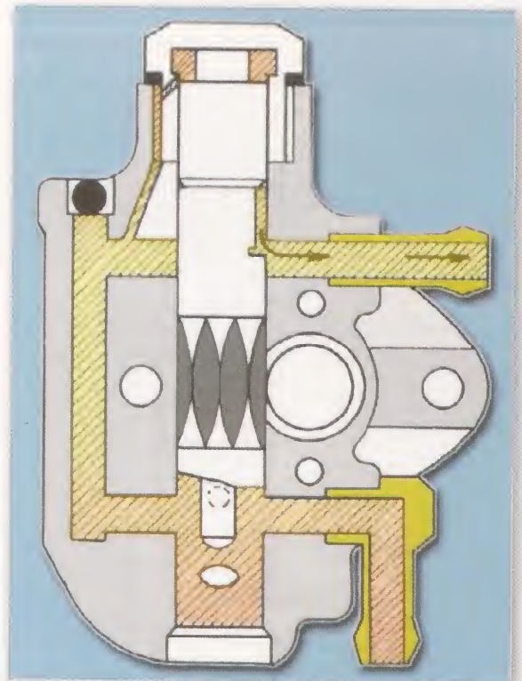
Flujo de aceite en corte de bomba autolube
